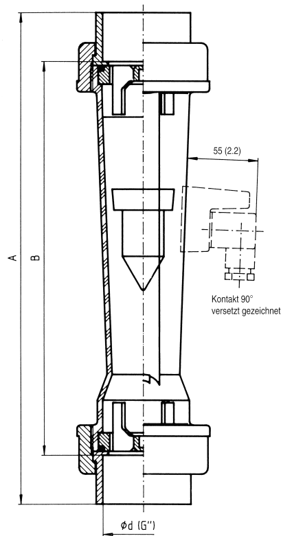
Abb. 4 Troglux Kurzbauf orm, Maße in mm
