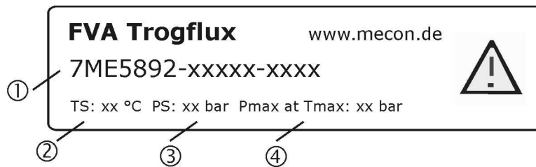
Abb. 3 Typenschild FVA Troglux Kurzbauforn
