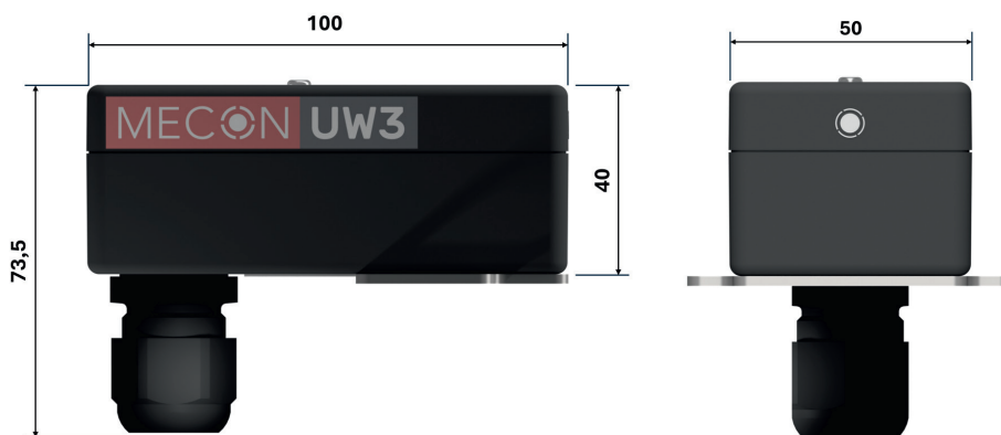
Abb. 1: Maße UW3 (mm)
