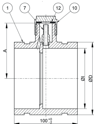
Abb. 2: Turbo-Lux® 3 Messblende, Positionszeichnung u. Maße für 2"/DN 50 ... 4"/DN 100
